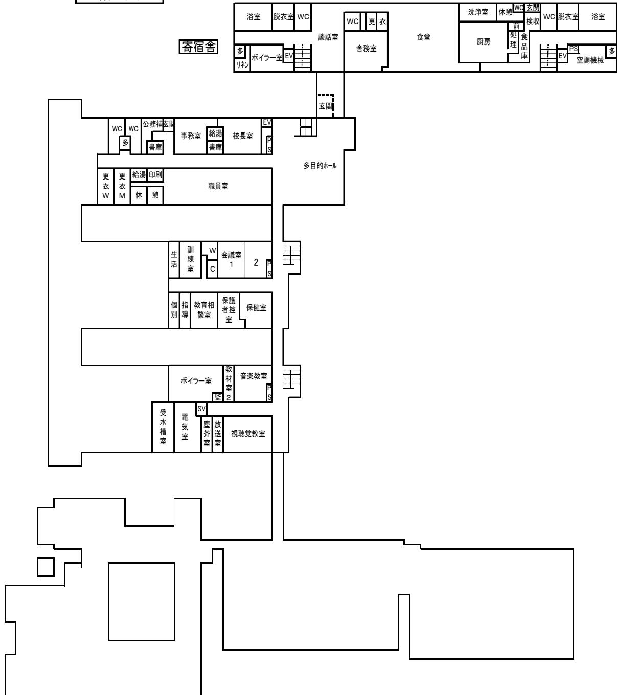
1階平面図
